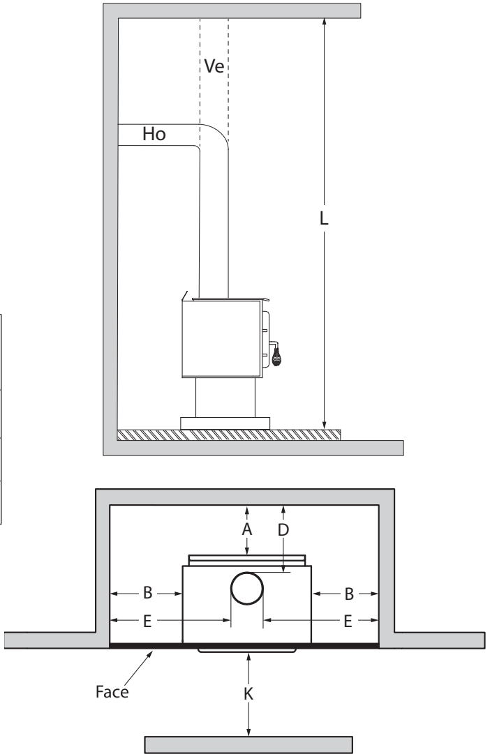
Figure 13: Dégagements - Alcôve
