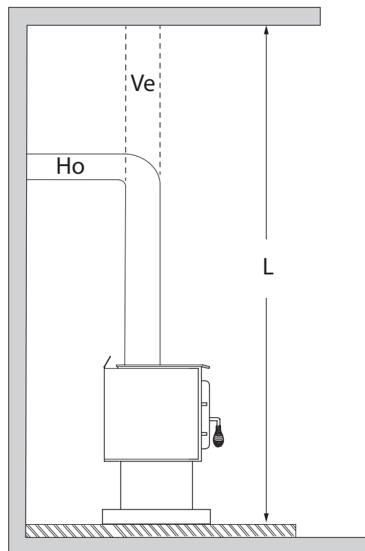
Figure 7: Dégagements - Plafond
