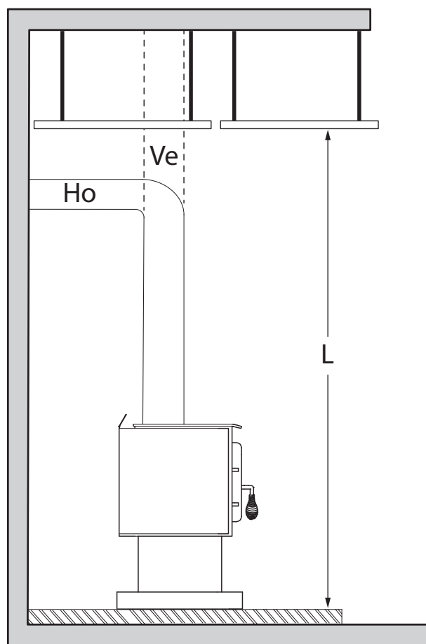
Figure 12: Dégagements - Plafond
