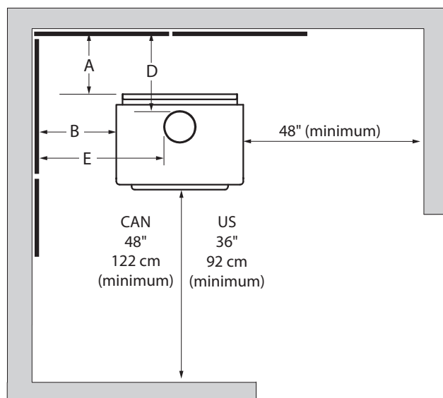
Figure 10: Dégagements - Vue dessus avec écran
