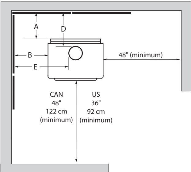
Figure 14: Dégagements - Vue dessus avec écran
