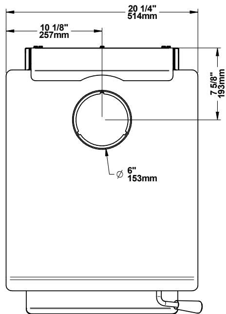
Figure 1: Vue de dessus
