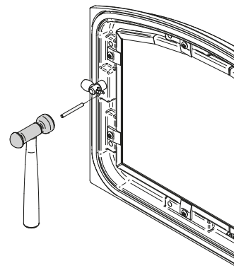
Figure 22: Installation de la goupille de retenue
