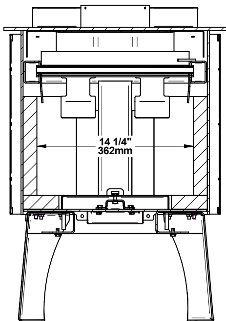
Figure 5: Vue de face - chambre à combustion
