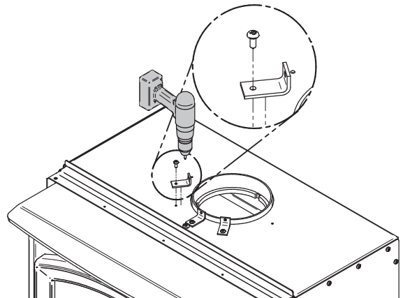
Figure 31: Installation des équerres
