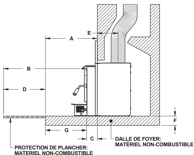
Figure 26: Protection de plancher aditionnelle - Installation non surélevée
