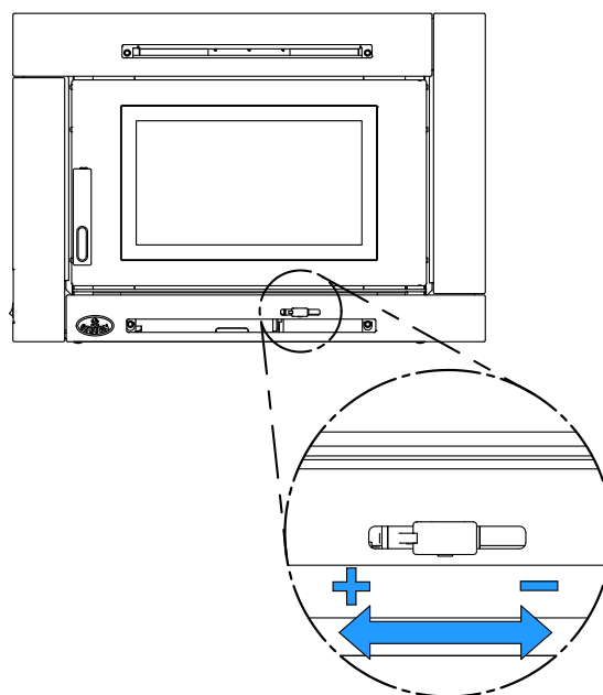
Figure 22: Contrôle de l'admission d'air
