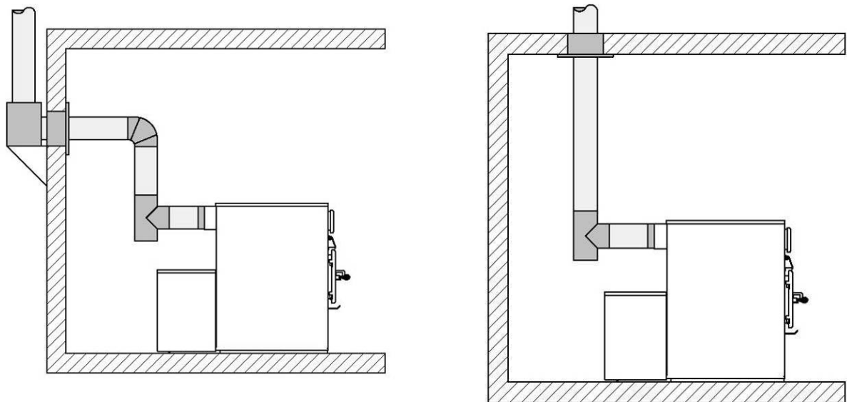
Installations alternatives avec coude 90° ou té.
