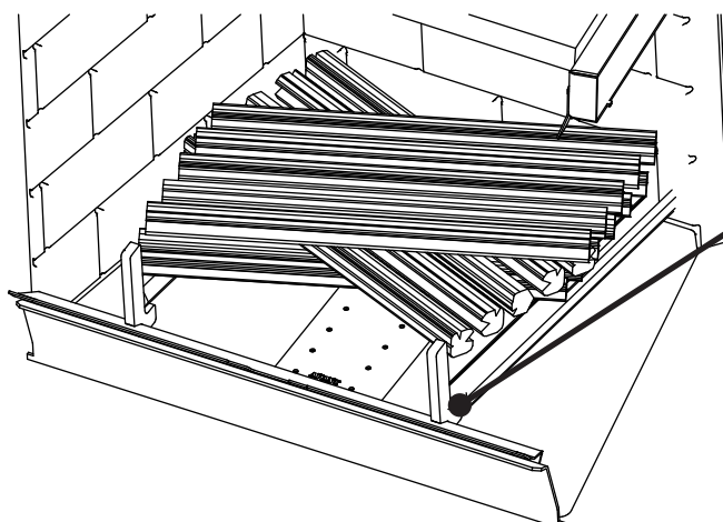
Figure 13: Configuration des allumettes utilisant l'améliorateur d'allumage des allumettes (KIE) - Vue du dessus
