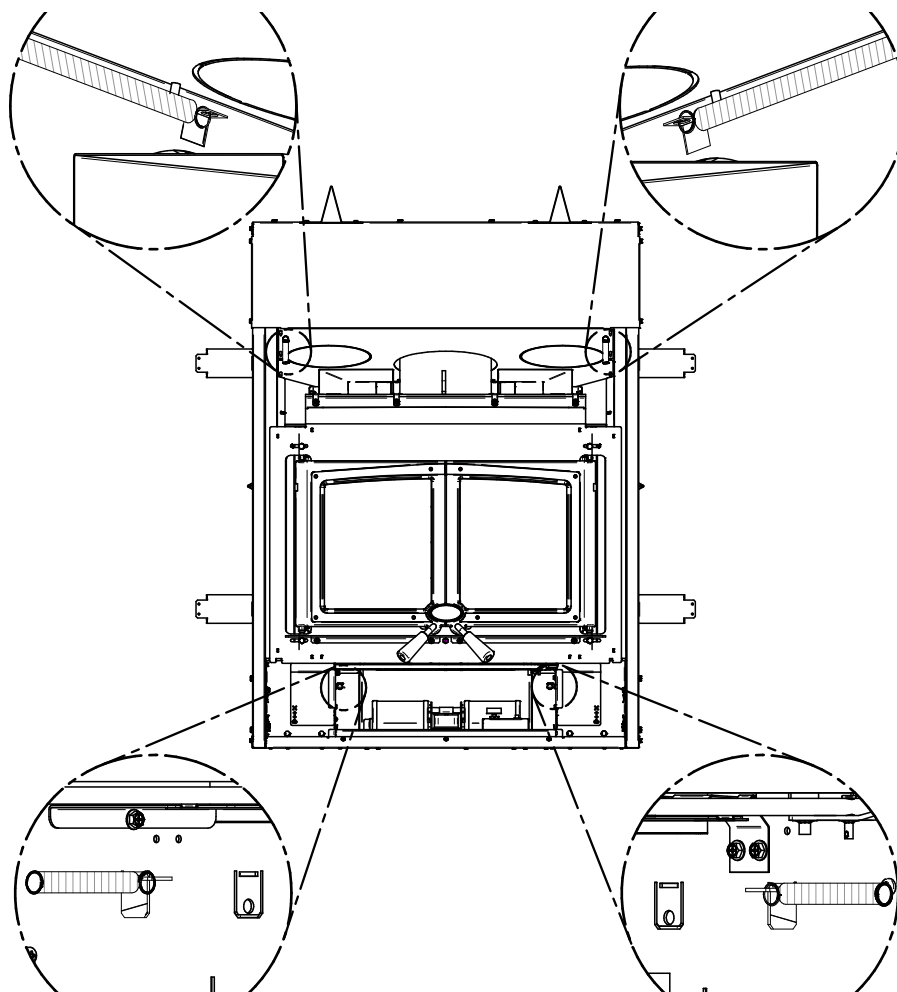
INSTALLATION DES RESSORTS (fournit avec le kit de manuel du produit)
