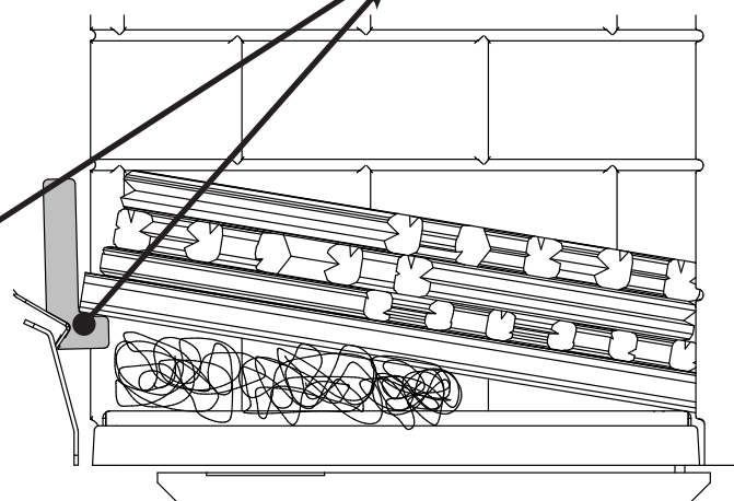
Figure 14: Configuration des allumettes utilisant l'améliorateur d'allumage des allumettes (KIE) - Vue de côté
