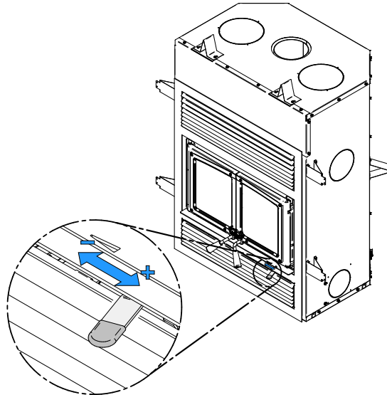
Figure 11: Commande d'air
