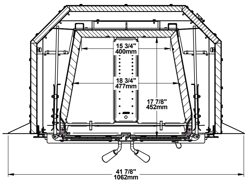
Figure 6: Chambre à combustion - Vue de dessus
