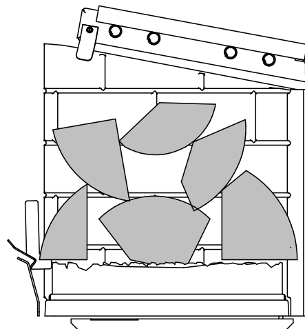
Figure 27: Configuration de charge à faible taux de combustion - Vue de côté
