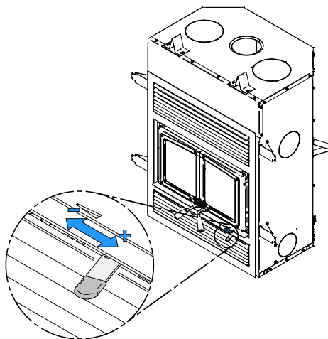
Figure 11: Commande d'air
