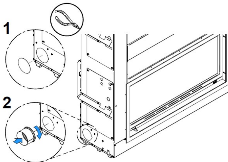
Figure 3 : Installation de l'adaptateur
