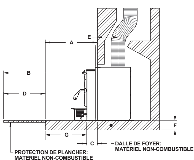
Figure 13: Protection de plancher additionnelle - Installation non surélevée
