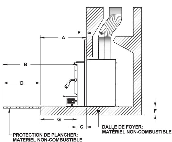
Figure 11: Protection de plancher aditionnelle - Installation non surélevée
