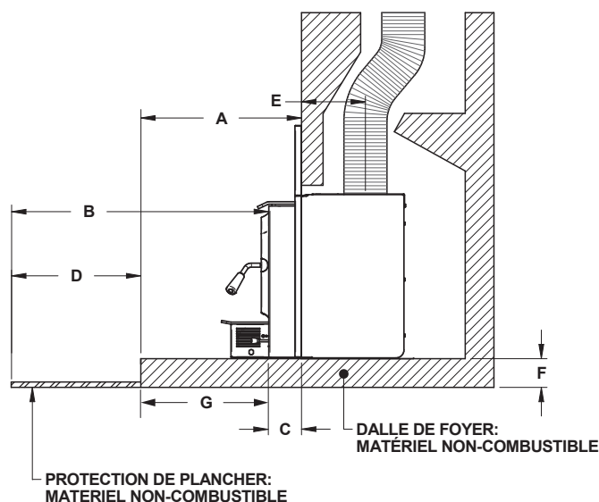
Figure 10: Protection de plancher aditionnelle - Installation surélevée
