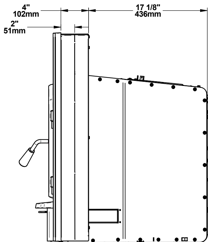
Figure 4: Vue de côté - Projection maximum
