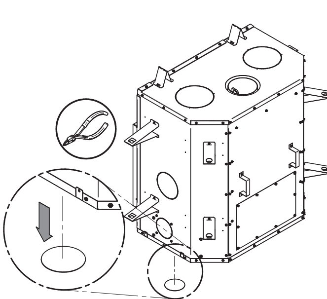
Figure 2: Entrée d'air sous le foyer
