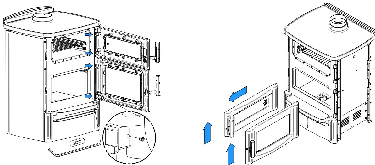
Figure 31: Libérer les pentures excentriques
