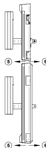
Figure 34: Ajustement en profondeur des pentures excentriques
