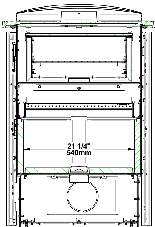
Figure 5: Vue de face - chambre à combustion
