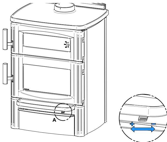
Figure 28: Contrôle de l'admission d'air
