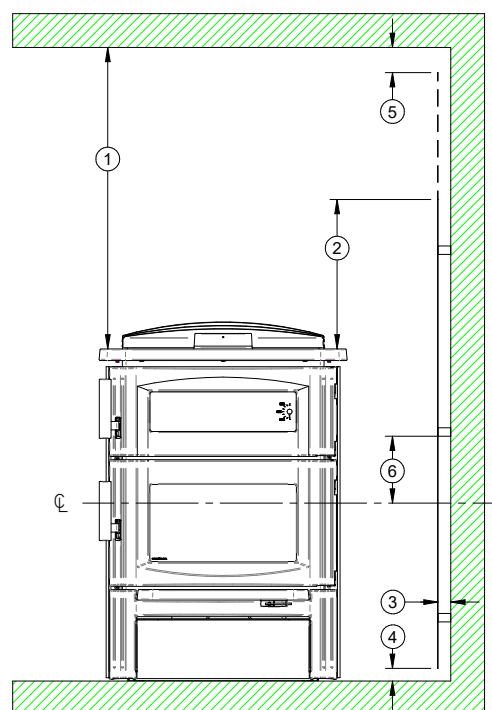
Figure 45: Dégagements avec écran mural - Face
