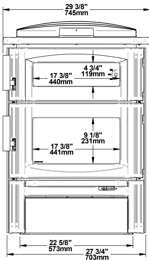
Figure 2: Vue de face
