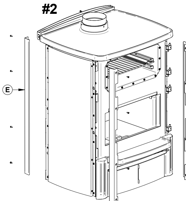
Figure 37: Retirer les moulures
