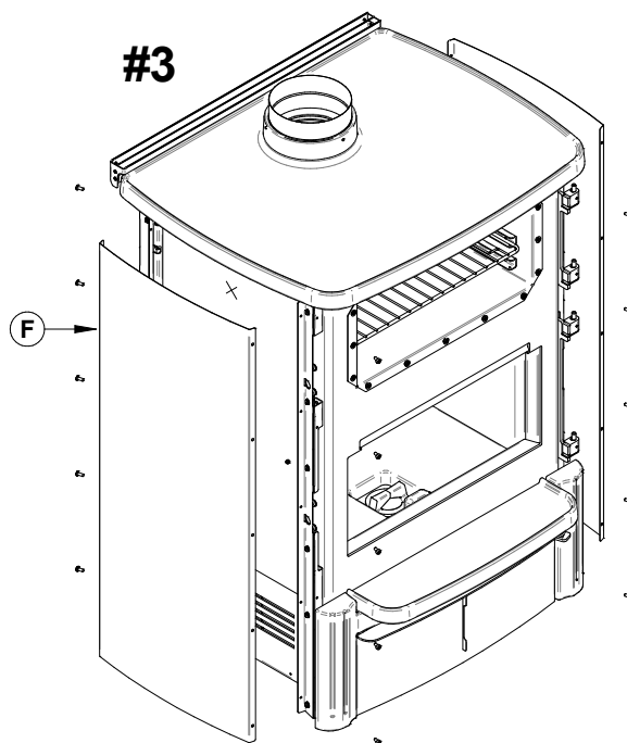
Figure 38: Retirer les panneaux décoratifs
