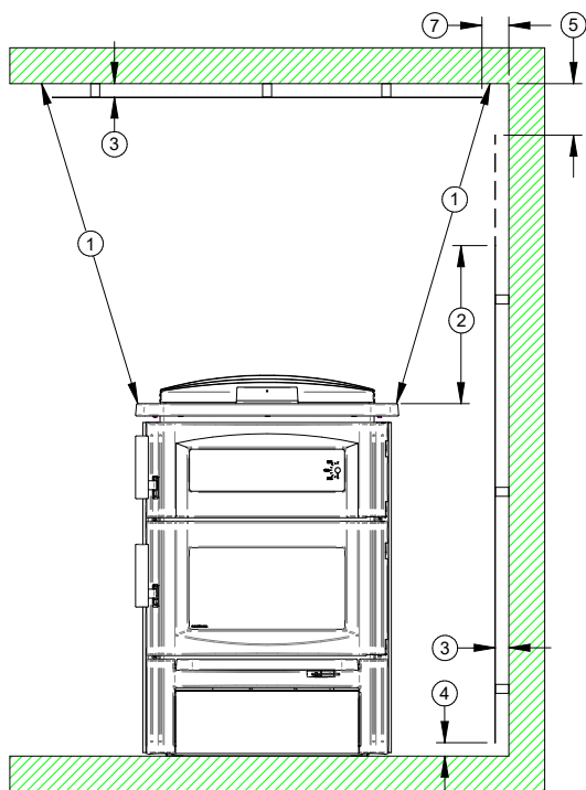
Figure 44: Dégagements avec écran mural - Face
