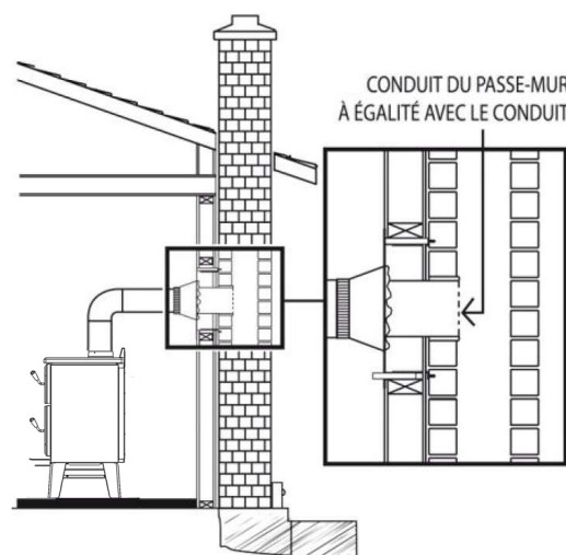
Figure 48: Installation dans un âtre de maçonnerie
