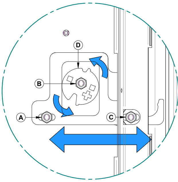
Figure 29: Ajustement porte de la chambre à combustion
