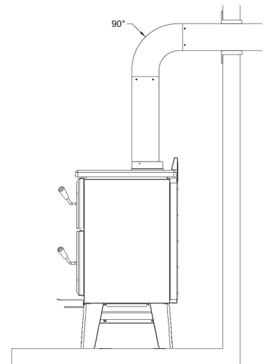
Figure 55: Éviter
