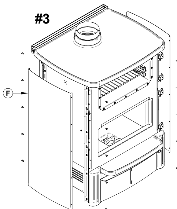
Figure 38: Retirer les panneaux décoratifs
