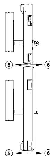
Figure 34: Ajustement en profondeur des pentures excentriques
