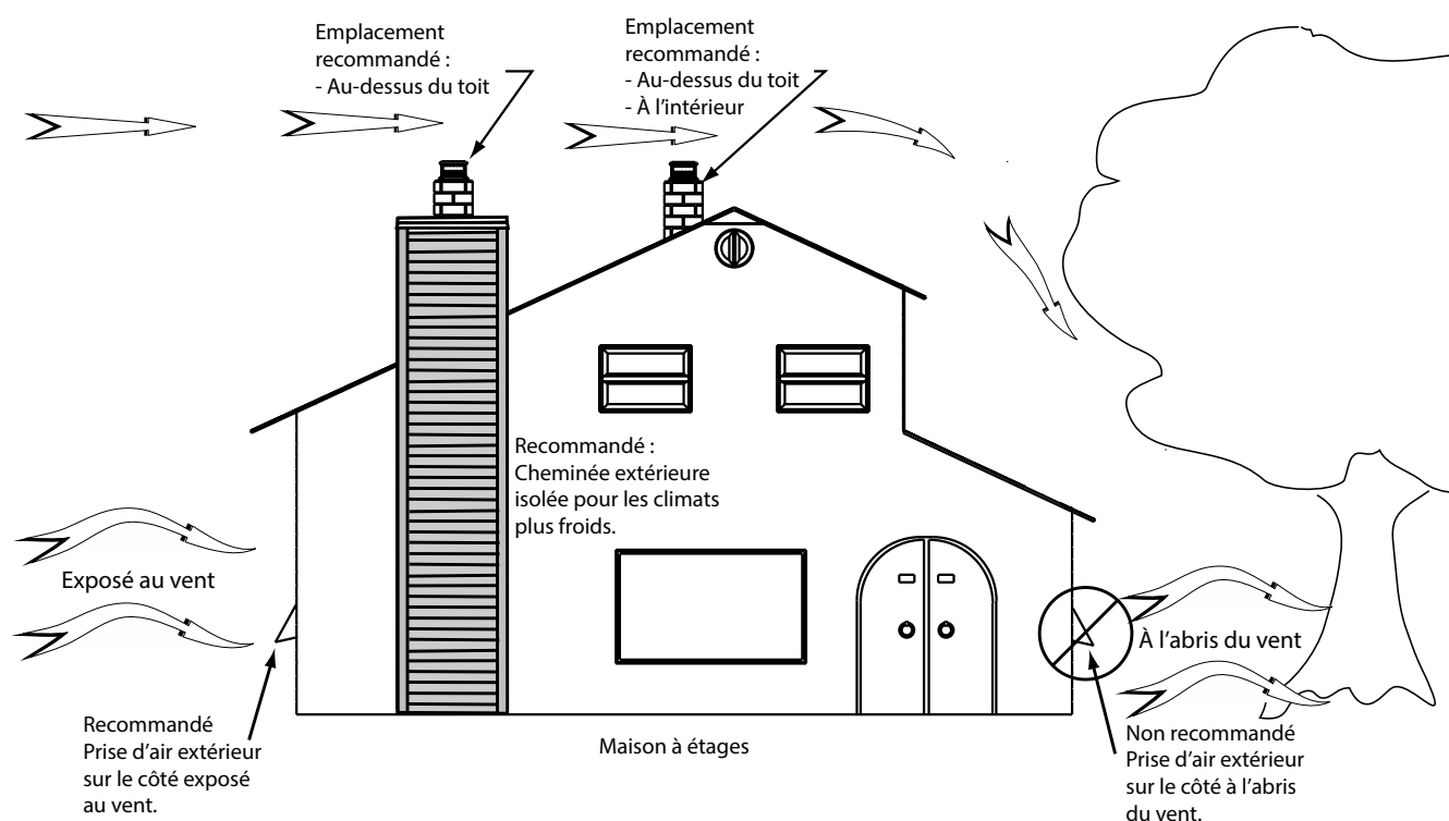
Figure 57: Apport d'air dans les maisons conventionnelles
