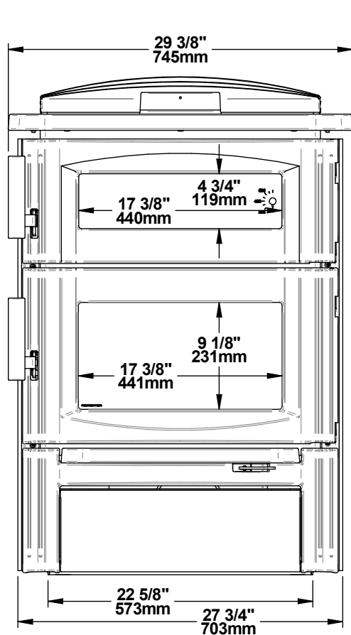
Figure 2: Vue de face
