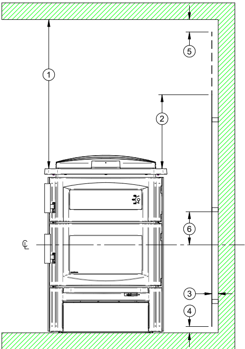
Figure 45: Dégagements avec écran mural - Face
