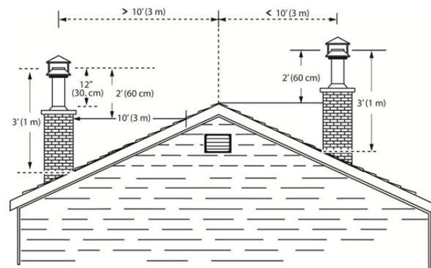
Figure 50: Toit en pente
