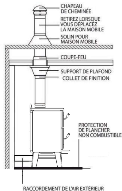
Figure 47: Installation en maison mobile
