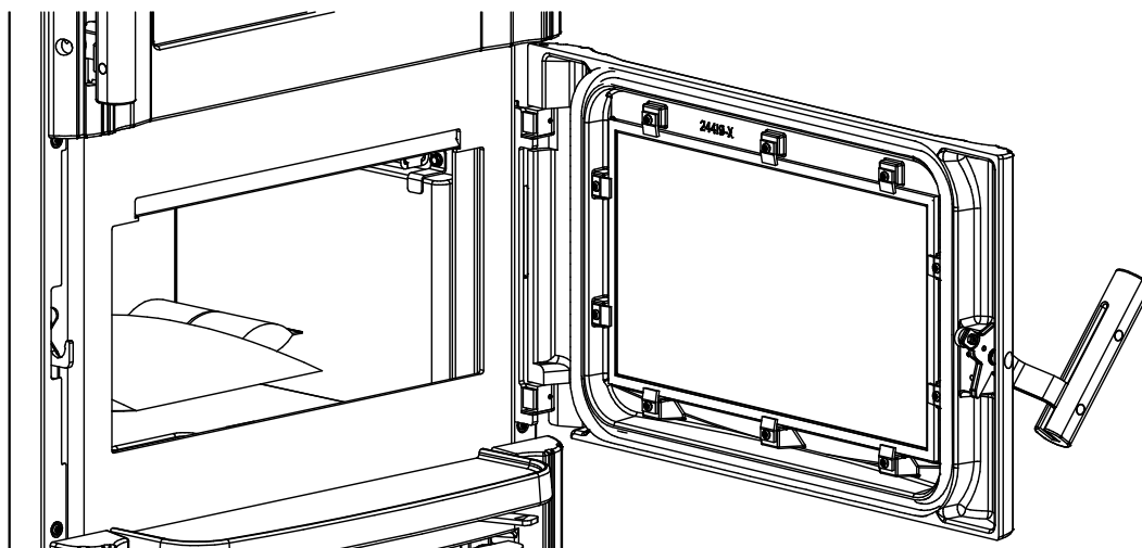
Figure 23: Chambre à combustion porte ouverte
