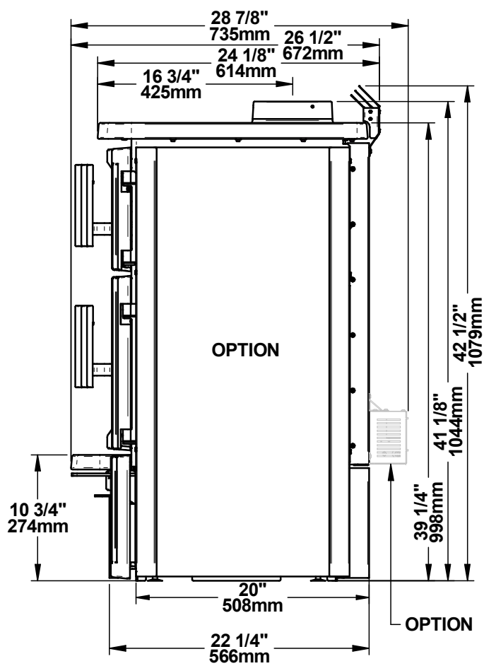
Figure 3: Vue de côté
