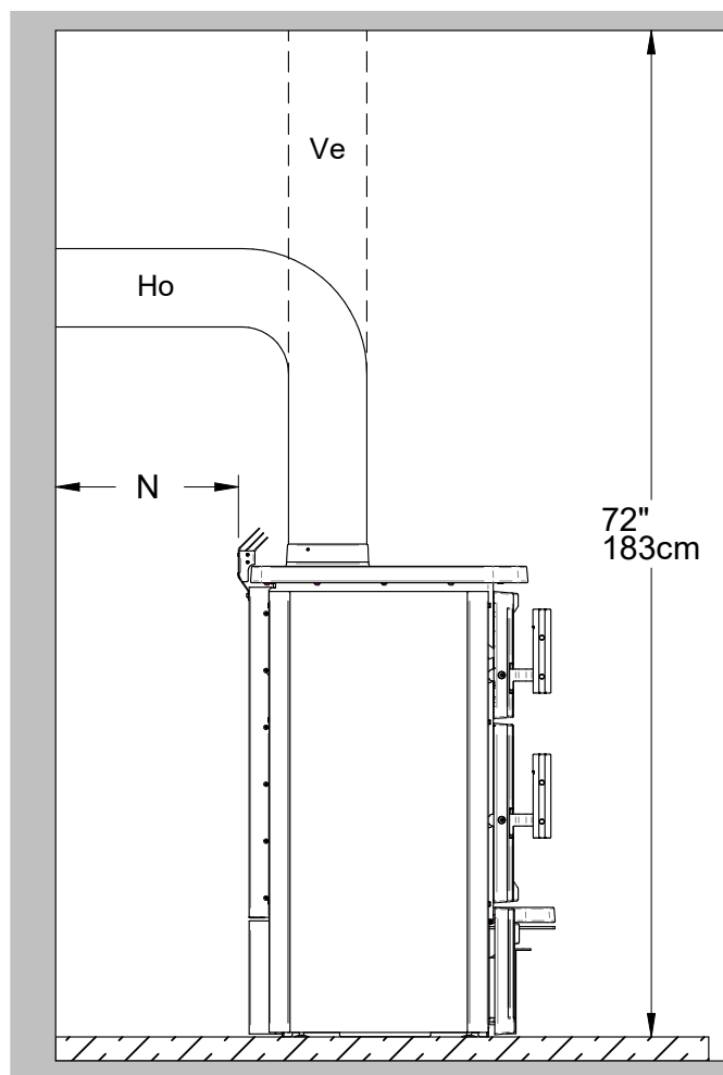
Figure 40: Dégagement au plafond
