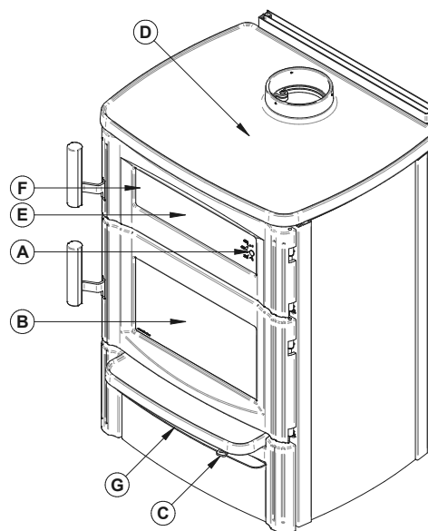
Figure 19: Localisation des composants
