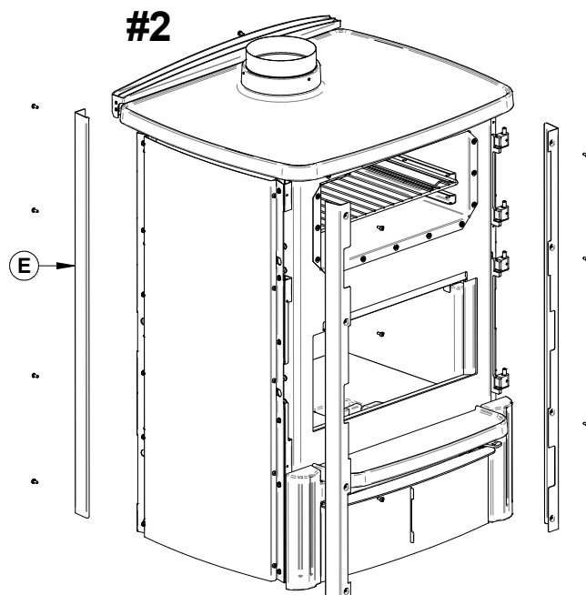
Figure 37: Retirer les moulures
