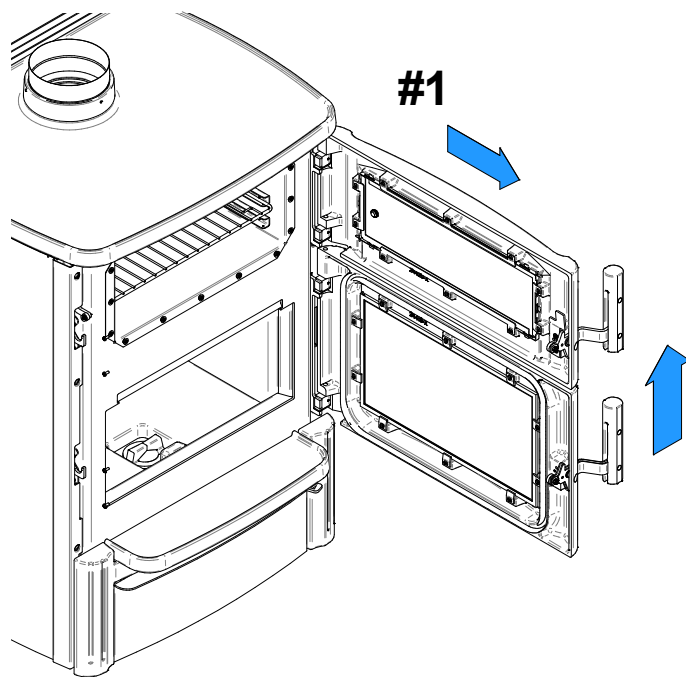
Figure 36: Enlever les portes
