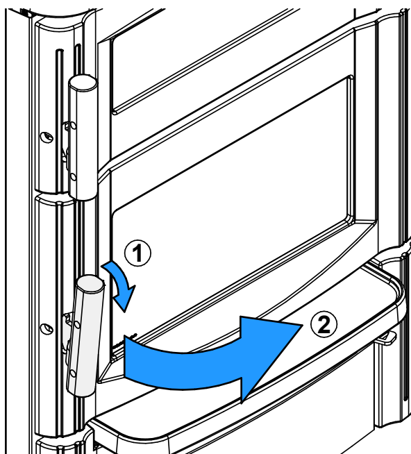
Figure 22: Chambre à combustion porte fermée
