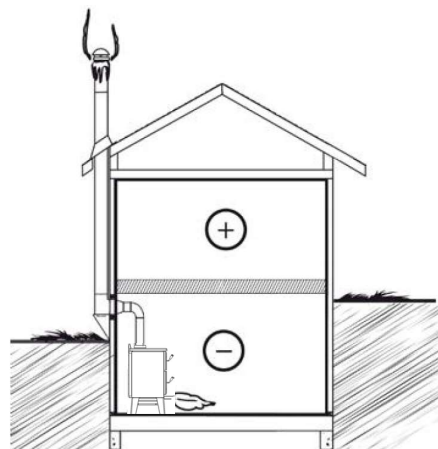
Figure 52: Conception de système acceptable
