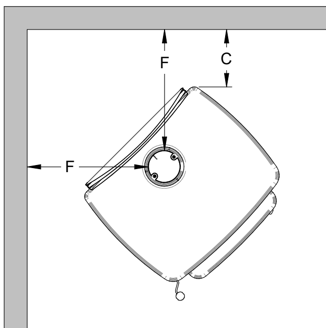
Figure 39: Dégagements aux murs adjacents
