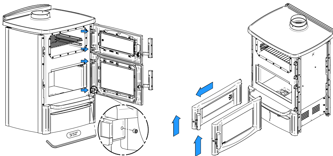
Figure 31: Libérer les pentures excentriques
