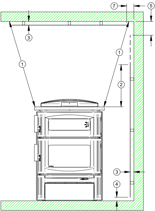
Figure 44: Dégagements avec écran mural - Face
