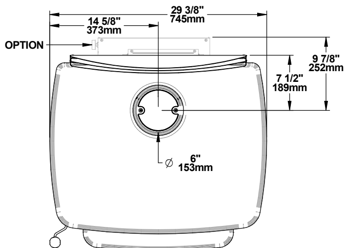
Figure 1: Vue de dessus
