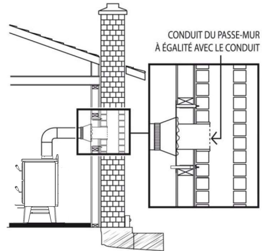
Figure 48: Installation dans un âtre de maçonnerie
