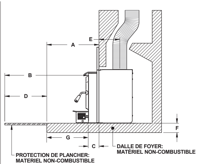
Figure 13: Protection de plancher additionnelle - Installation non surélevée
