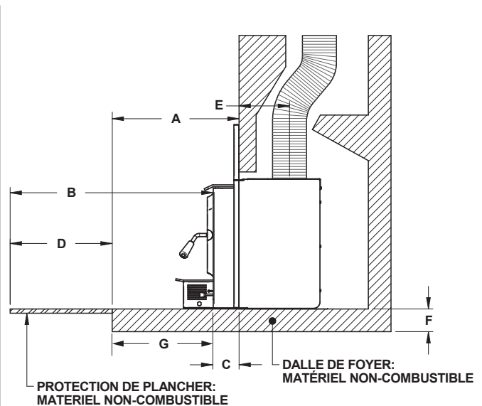
Figure 11: Protection de plancher aditionnelle - Installation non surélevée
