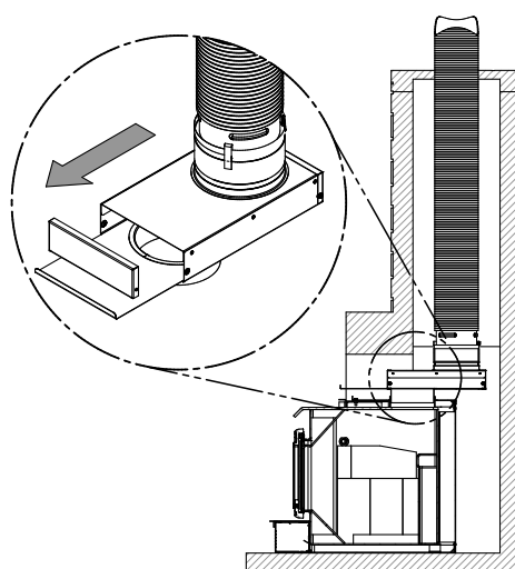
Figure 20: Adaptateur de déviation de gaine
