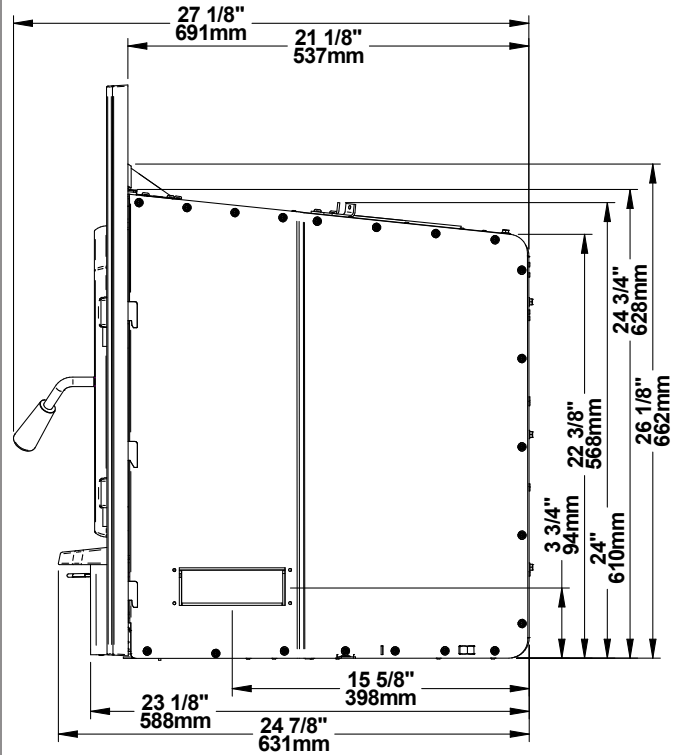
Figure 2: Vue de côté - Projection minimum
