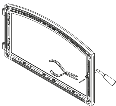
Figure 8: Retrait de la goupille de retenue
