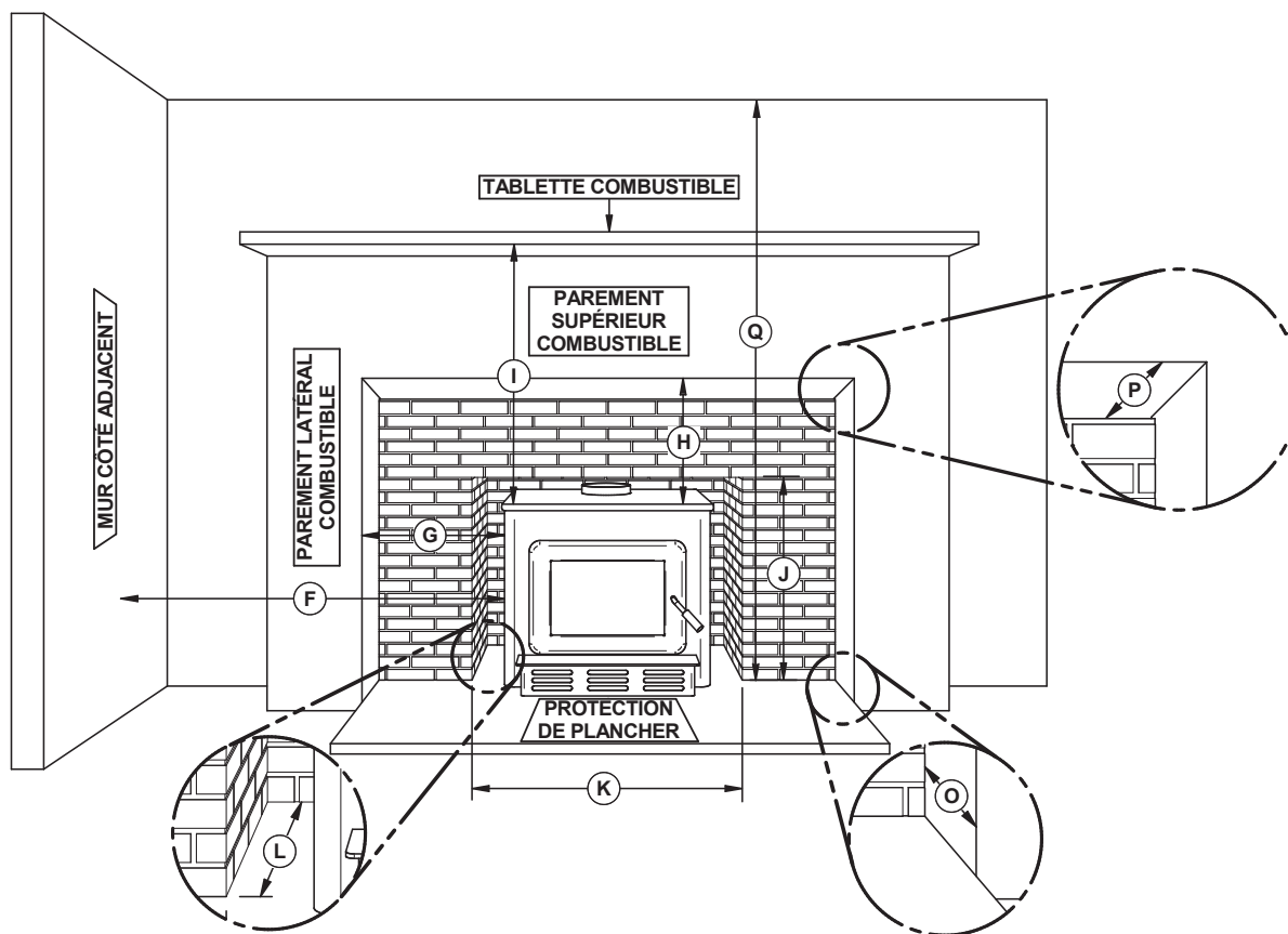
Figure 32: Ouverture de l'âtre et dégagements aux combustibles
