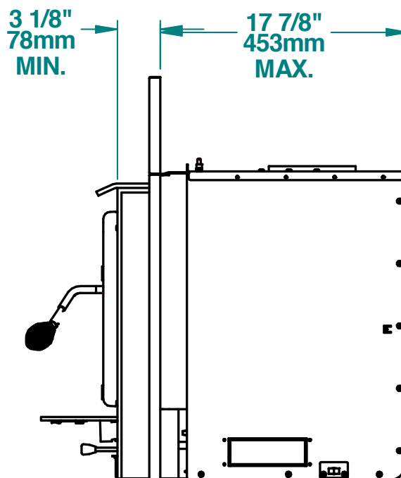
Figure 2: Vue de côté - Projection minimum
