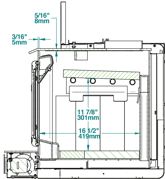
Figure 6: Vue de côté - Chambre à combustion
