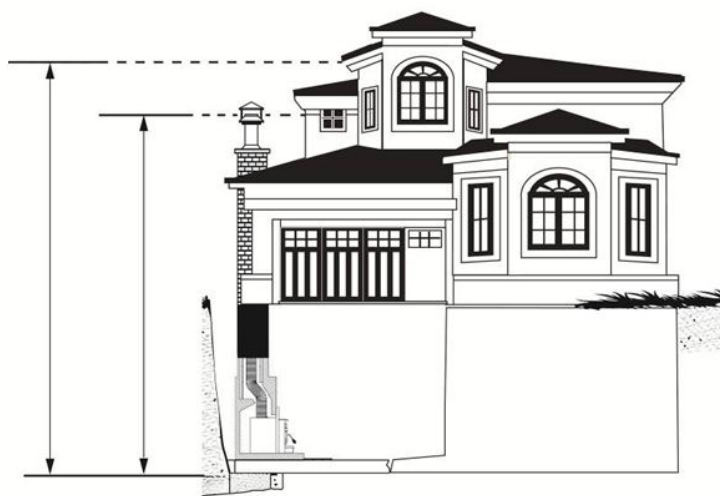
Figure 41: Positionnement de la cheminée dans l'habitation
