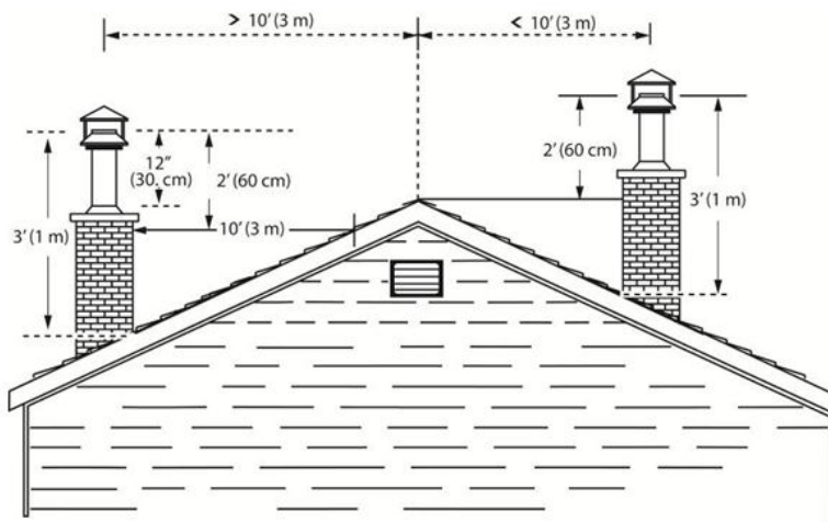
Figure 40: Hauteur minimale de la cheminée
