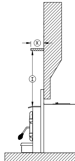
Figure 27: Dégagement de la tablette
