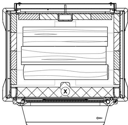
Figure 17: Position des bûches du bas (Taux de combustion moyen)
