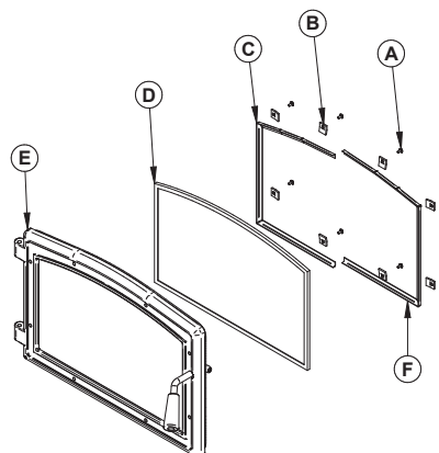
Figure 25: Remplacement de la vitre
