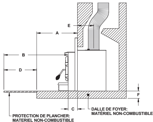
Figure 30: Installation surélevée de 5" ou moins
