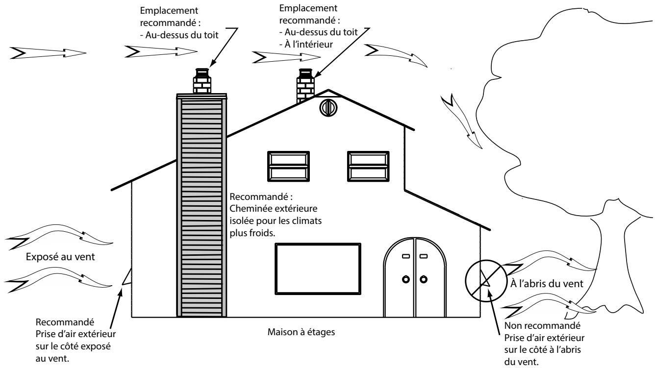
Figure 42: Positionnement de l'entrée d'air frais
