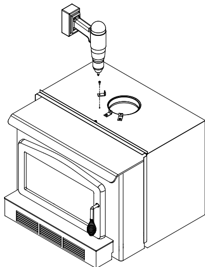
Figure 36: Équerres de fixation
