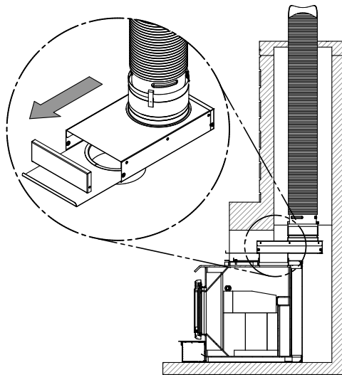
Figure 39: Adaptateur de déviation de gaine
