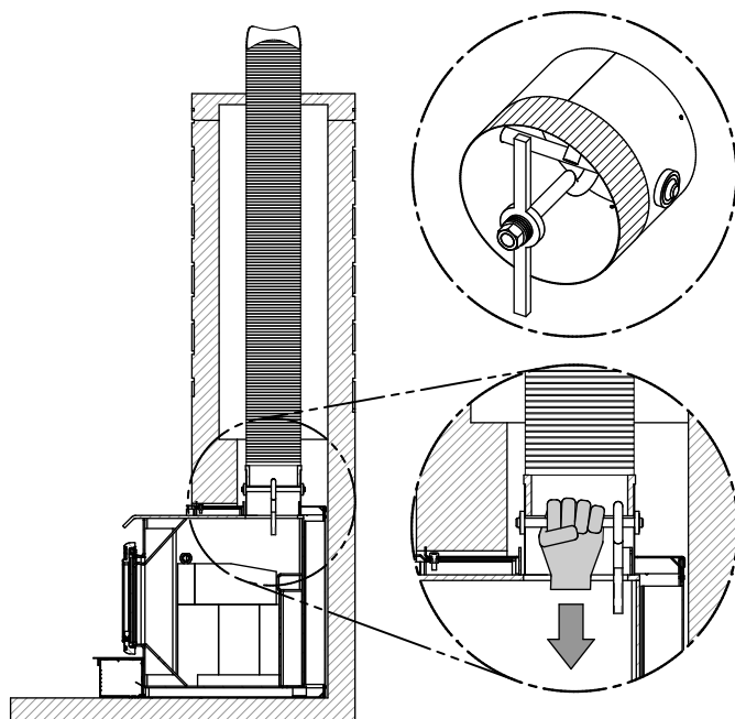
Figure 37: Système d'attache pour gaine
