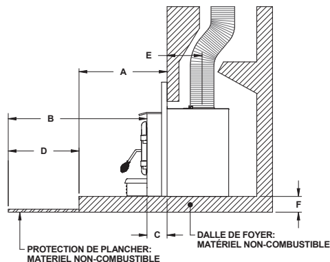
Figure 31: Installation surélevée de plus de 5"
