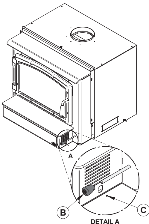
Figure 20: Bouton de la tige du contrôle d'air (B)
