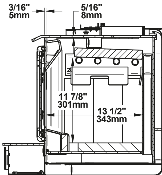
Figure 7 : Vue de côté - Chambre à combustion
