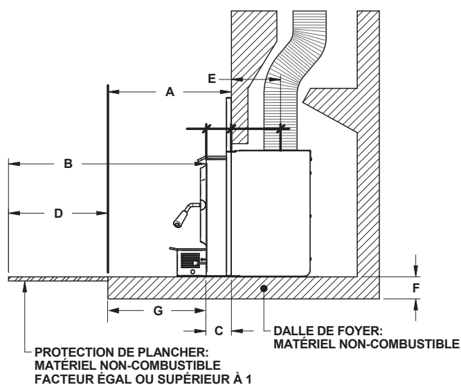
Figure 9 : Protection de plancher aditionnelle - Installation non surélevée
