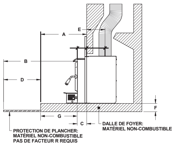
Figure 8 : Protection de plancher aditionnelle - Installation surélevée
