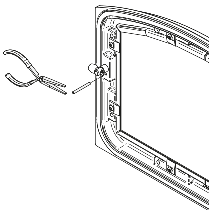
Figure 10 : Retrait de la goupille de retenue
