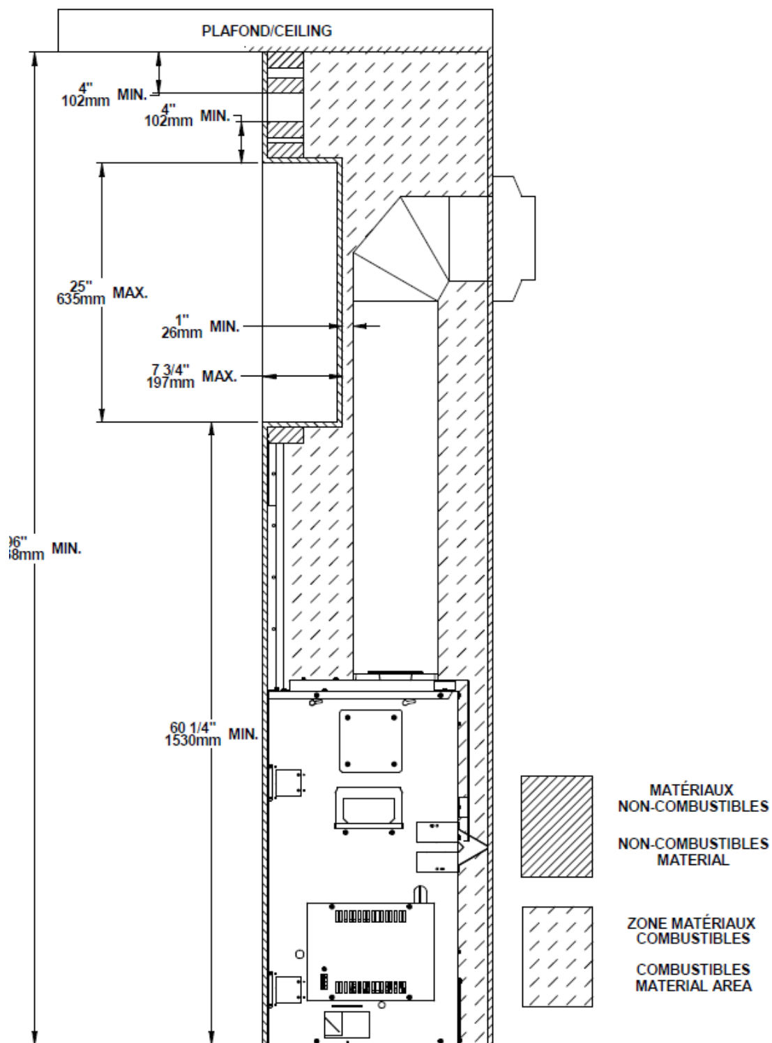
Figure 3 : Emplacement de la grille d'aération avec alcôve pour téléviseur
