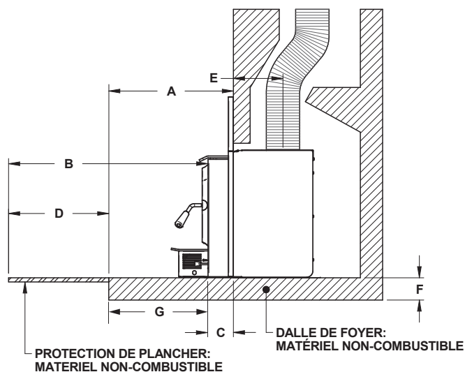
Figure 8 : Protection de plancher aditionnelle - Installation non surélevée
