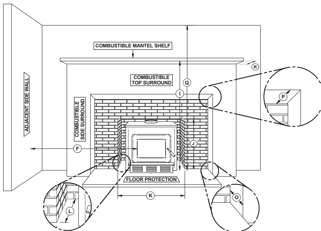
Figure 14 : Ouverture de l'âtre et dégagements aux combustibles
