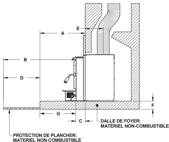
Figure 7 : Protection de plancher aditionnelle - Installation surélevée
