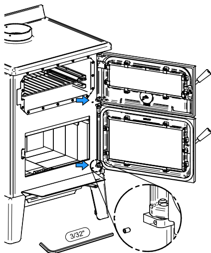
Figure 15: Libérer les pentures excentriques
