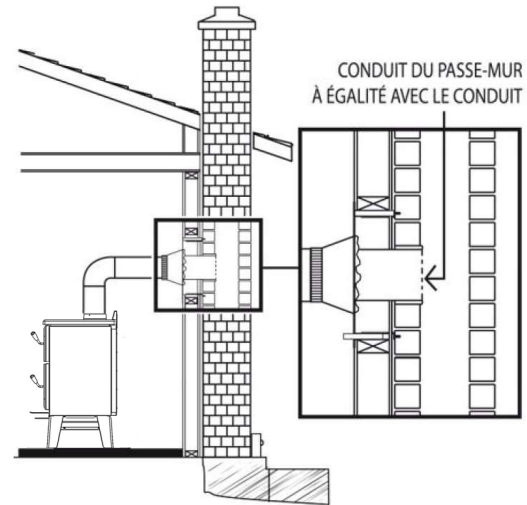
Figure 32: Installation dans un âtre de maçonnerie
