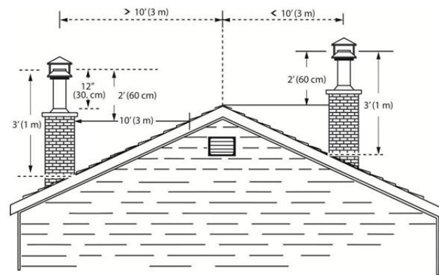
Figure 34: Toit en pente
