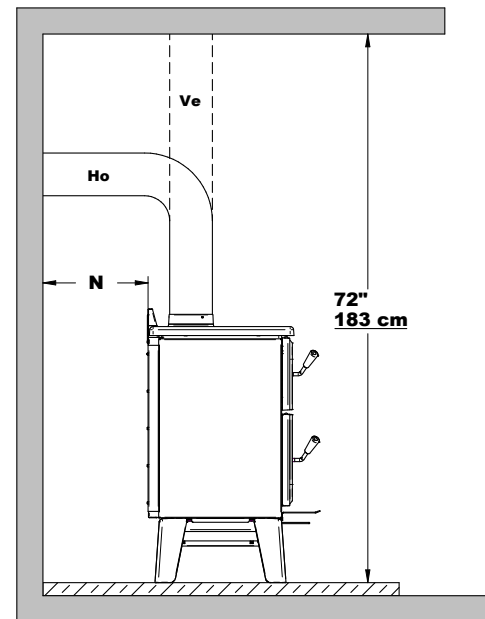
Figure 26: Dégagements
