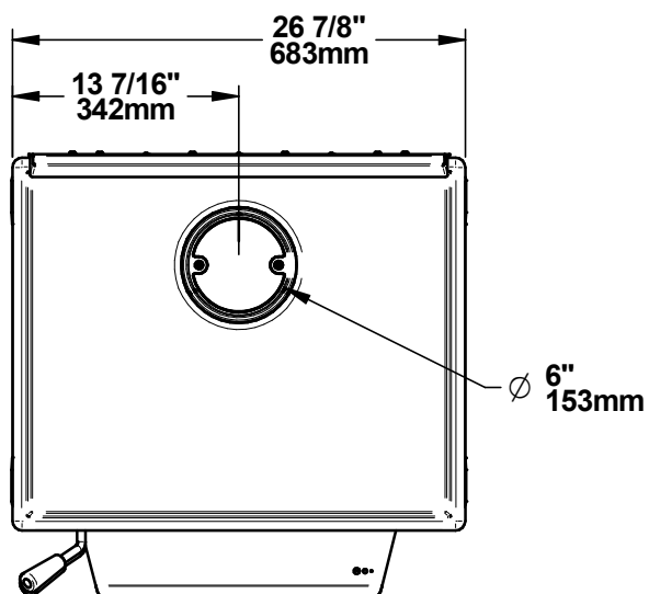
Figure 1: Vue de dessus
