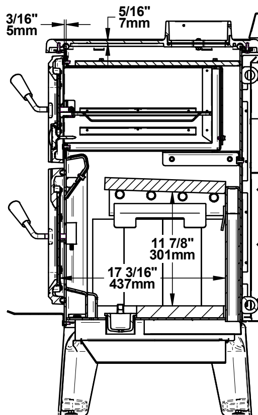
Figure 6: Vue de côté - chambre à combustion
