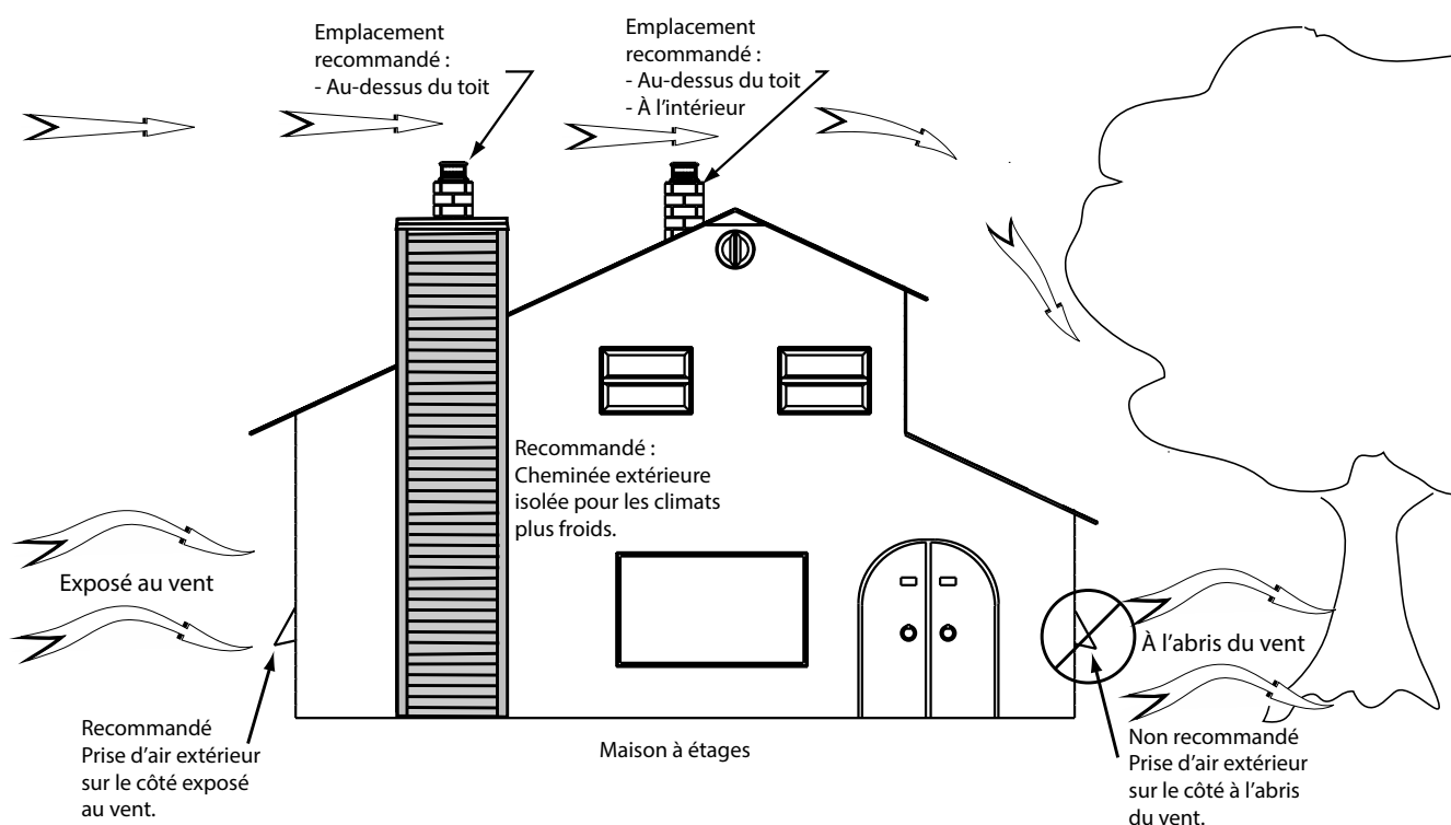
Figure 41: Apport d'air dans les maisons conventionnelles
