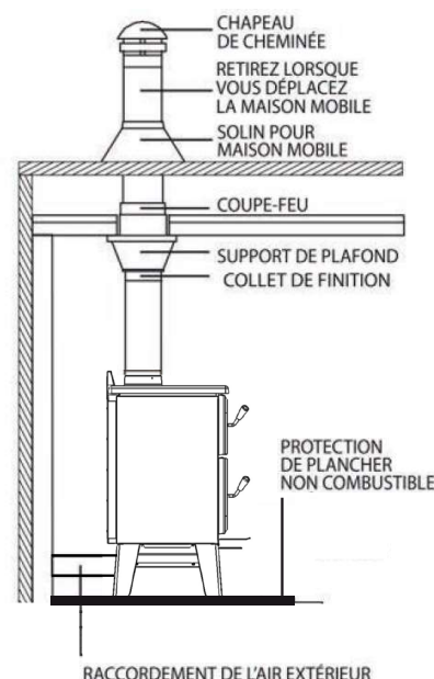
Figure 31: Installation en maison mobile
