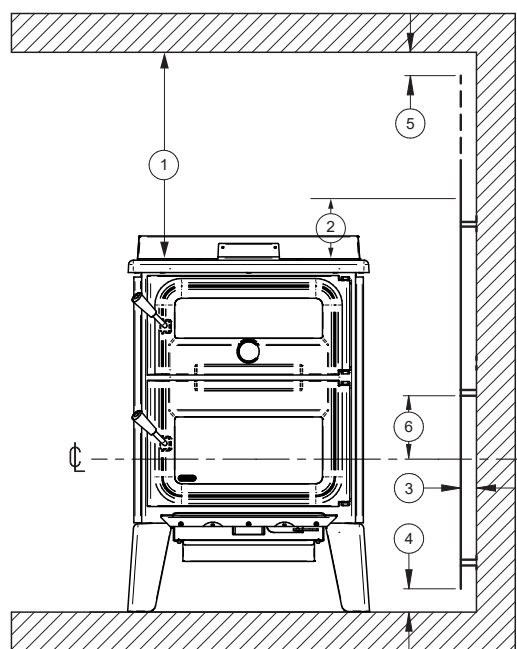
Figure 29: Dégagements avec écran mural - Face
