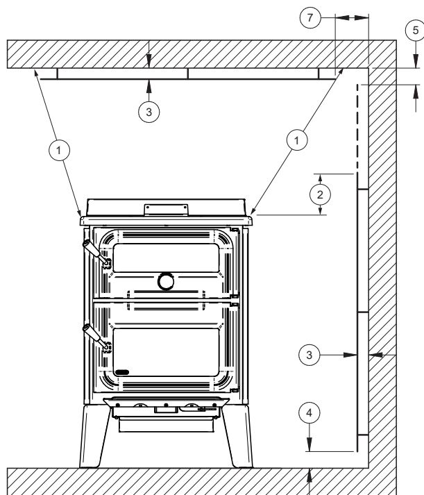
Figure 28: Dégagements avec écran mural - Face
