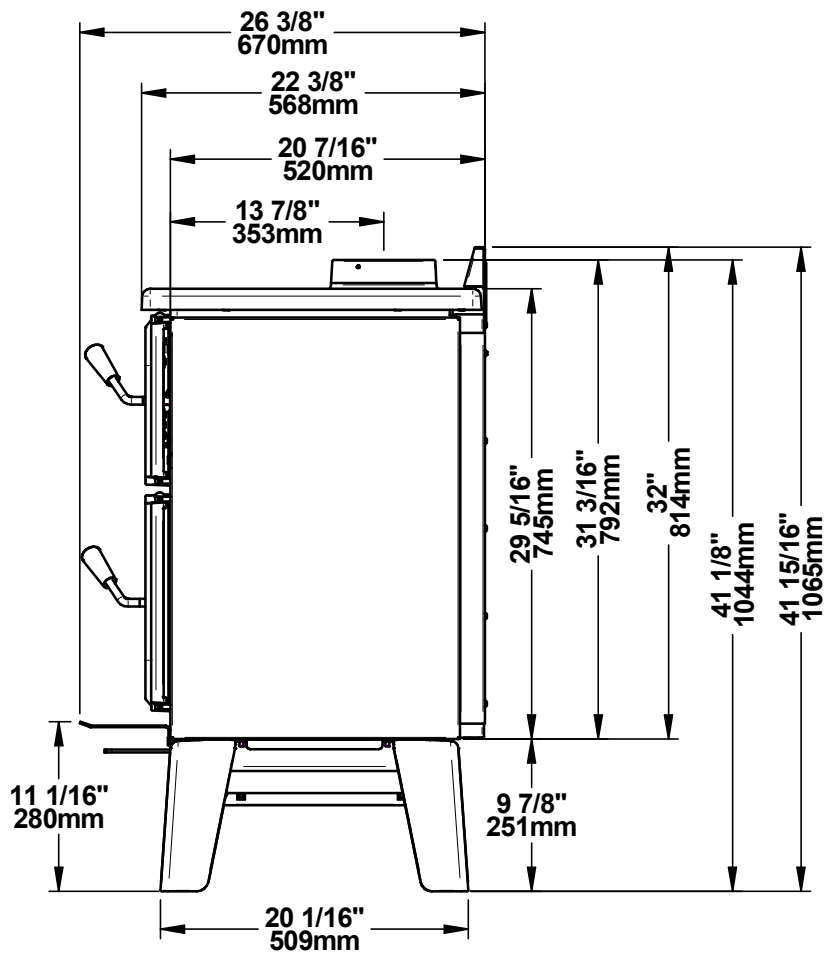
Figure 3: Vue de côté
