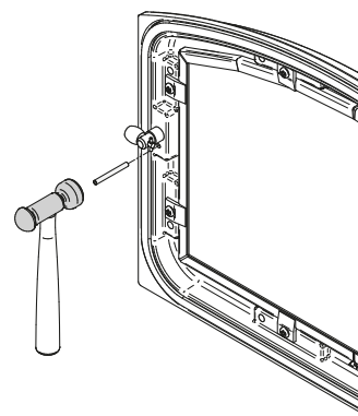
Figure 14: Installation de la goupille de retenue
