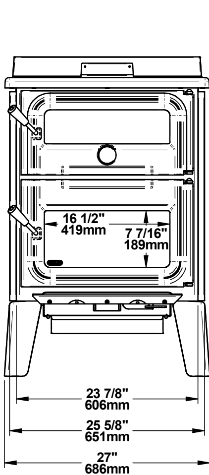
Figure 2: Vue de face
