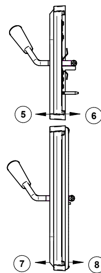
Figure 19: Ajustement en profondeur des pentures excentriques
