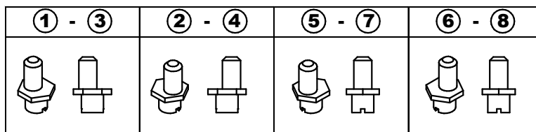
Figure 17: Ajustement latéral des pentures excentriques
